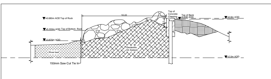
12 SECTION-27 1 : 100
