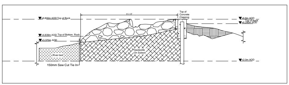
10 SECTION-26 1 : 100
