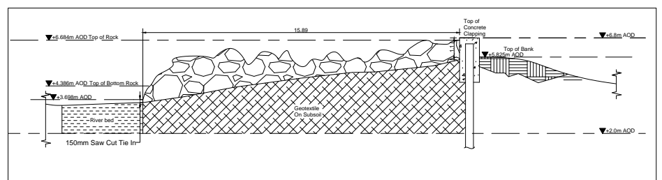
8 SECTION-24 1 : 100
