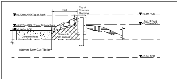
13 SECTION-19 1 : 100
