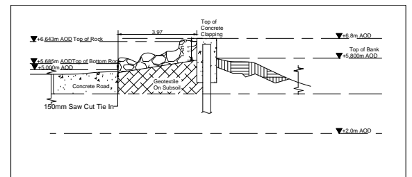
5 SECTION-21 1 : 100
