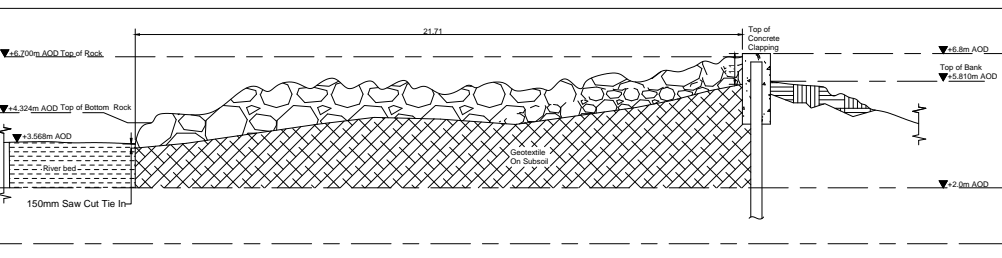
7 SECTION-23 1 : 100
