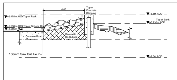
6 SECTION-22 1 : 100
