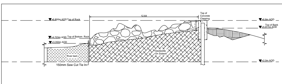
9 SECTION-25 1 : 100
