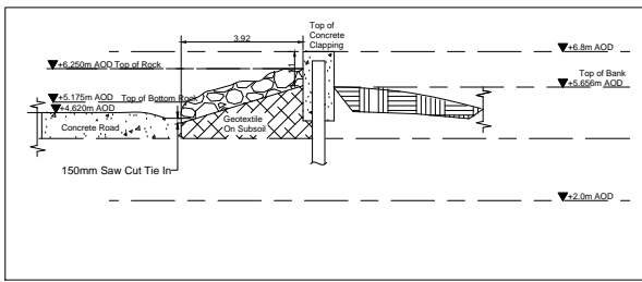
1 SECTION-16 1 : 100
