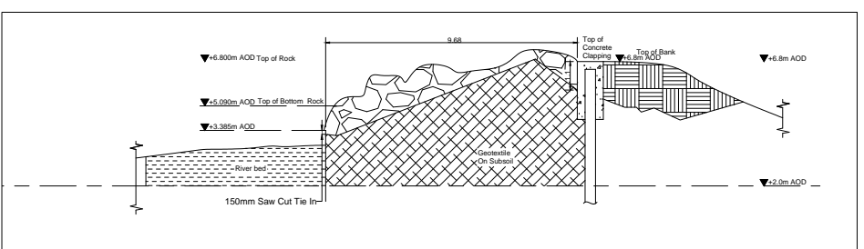
11 SECTION-28 1 : 100
