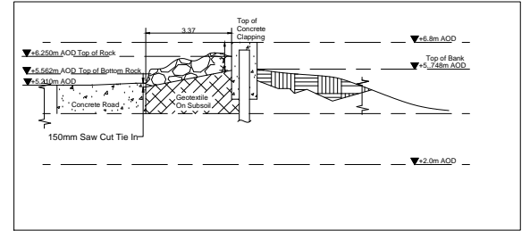
3 SECTION-18 1 : 100
