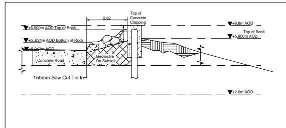
4 SECTION-20 1 : 100
