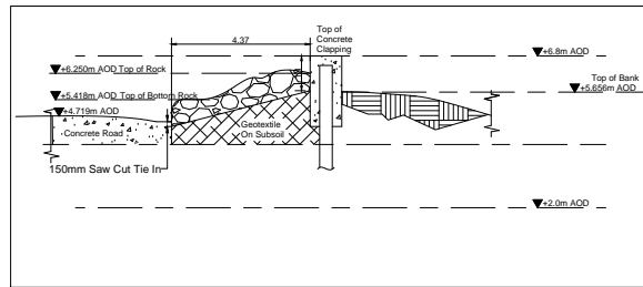
2 SECTION-17 1 : 100
